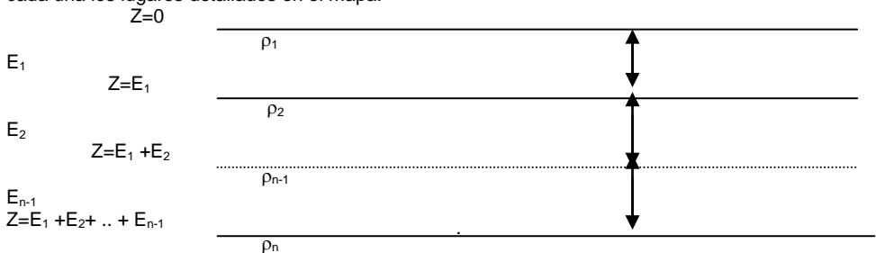
Figura 1 Modelo Geoelectrico unidimensional de una de serie de capas paralelas e isotropas
